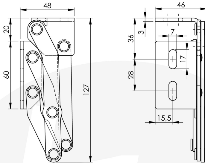
Abbildung Scharnier rechts Typ I
